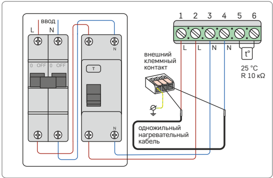
Схема 1. Схема подключения одножильного нагревательного кабеля к терморегулятору
