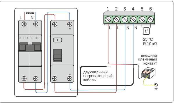
Схема 2. Схема подключения двухжильного нагревательного кабеля к терморегулятору
