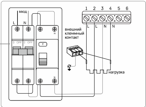
Схема 1. Схема подключения терморегулятора, автоматического выключателя, УЗО и нагревателя
